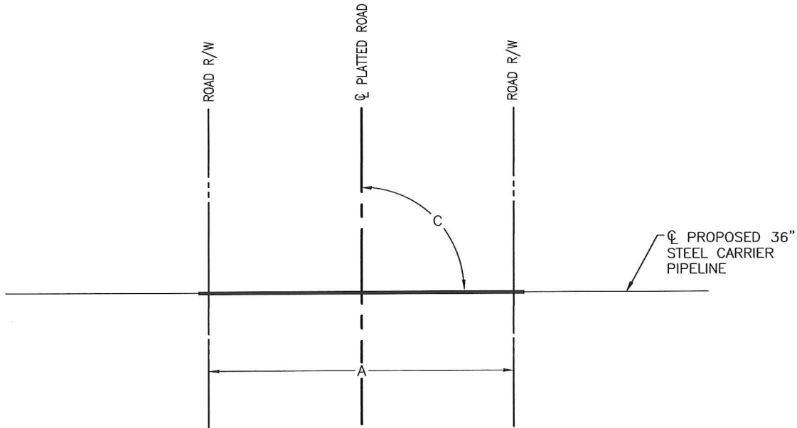
PLAN N.T.S.
