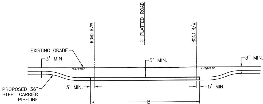
PROFILE N.T.S.
